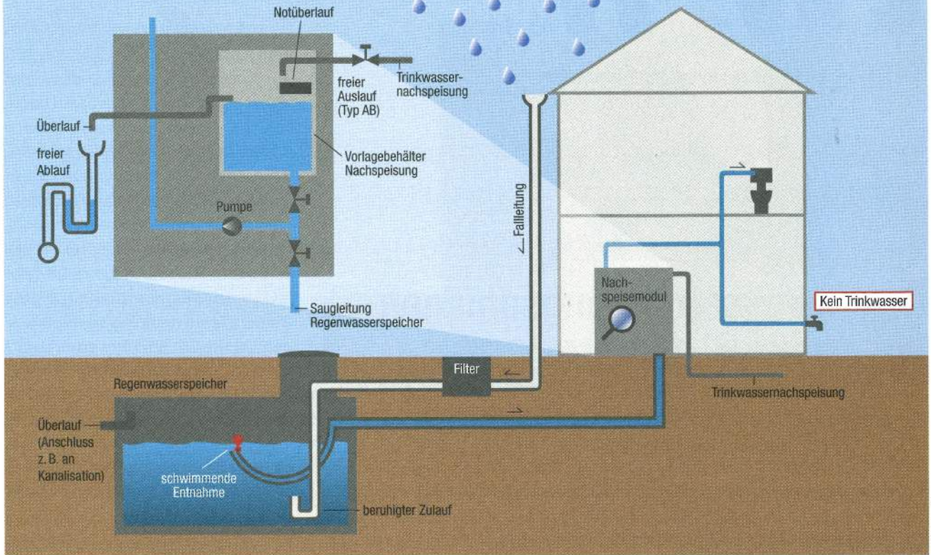
Abbildung 1: Einbau des freien Auslaufes zwischen Regenwassernutzungsanlage und Trinkwassernachspeisung (dargestellt ist der freie Auslauf Typ AB; möglich ist auch der Typ AA und AD, siehe DIN EN 1717)
