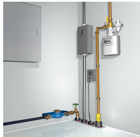
Unterbodeneinführung eckig für Gebäude ohne Keller
